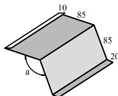
Фартук S11 на излом развертка 20см, длина 4(2)м
