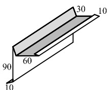
Фартук S5 фронтонный развертка 20см, длина 4(2)м
