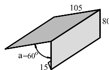
Фартук S16 обратный капельник развертка 20см, длина 4(2)м
