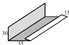
Фартук S9 вспомогательный развертка 10см, длина 2м
