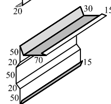
Фартук S7 пристенный в штрабу развертка 12,5см, длина 4(2)м
