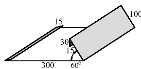
Фартук S12 разжелобка развертка 46см, длина 2м
