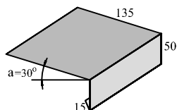
Фартук S14 карнизный над желобом развертка 20см, длина 2м
