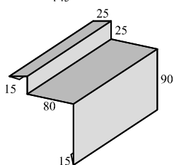
Фартук S20 пристенного аэратора в штрабу развертка 25см, длина 4(2)м
